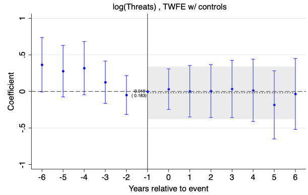
(d) log(threats)
